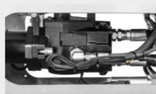
Motor hidráulico variable de pistones de 17/34 cc con desplazamiento de ajuste manual y con válvula de alivio y anti cavitación
