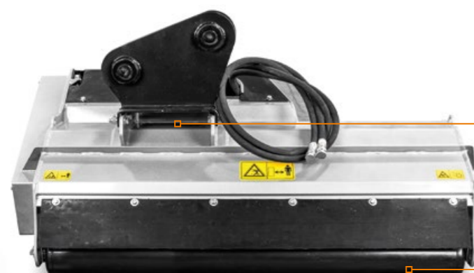
Rodillo posterior con dispositivo de auto limpieza
